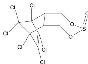
β-endosulfan (β-ES)
