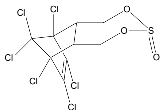
α-endosulfan (α-ES)
