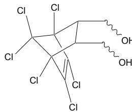
endosulfan diol (ES diol)
